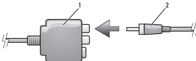
1 προσαρμογέας composite video 2 καλώδιο ψηφιακού ήχου S/PDIF video
